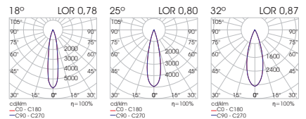
Antiglare Ring
